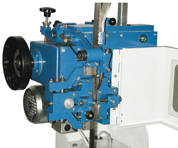
Gruppo testa Main setting head Schränkkopf
